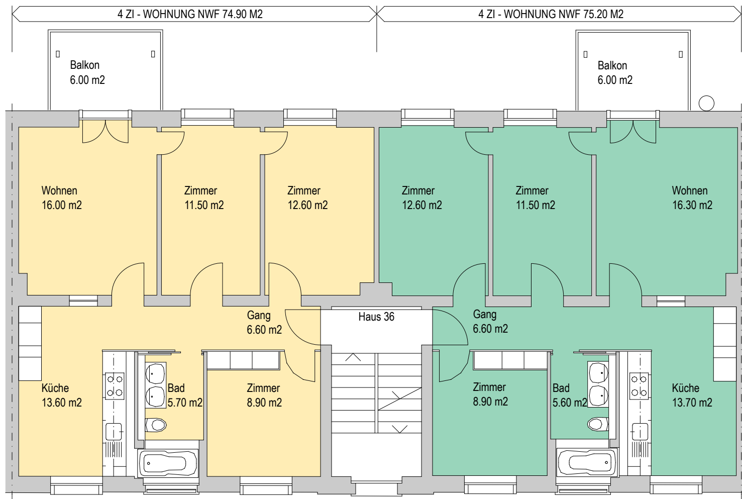
1. - 4. OBERGESCHOSS 1 : 100 NWF = NETTWOHNFLÄCHE
