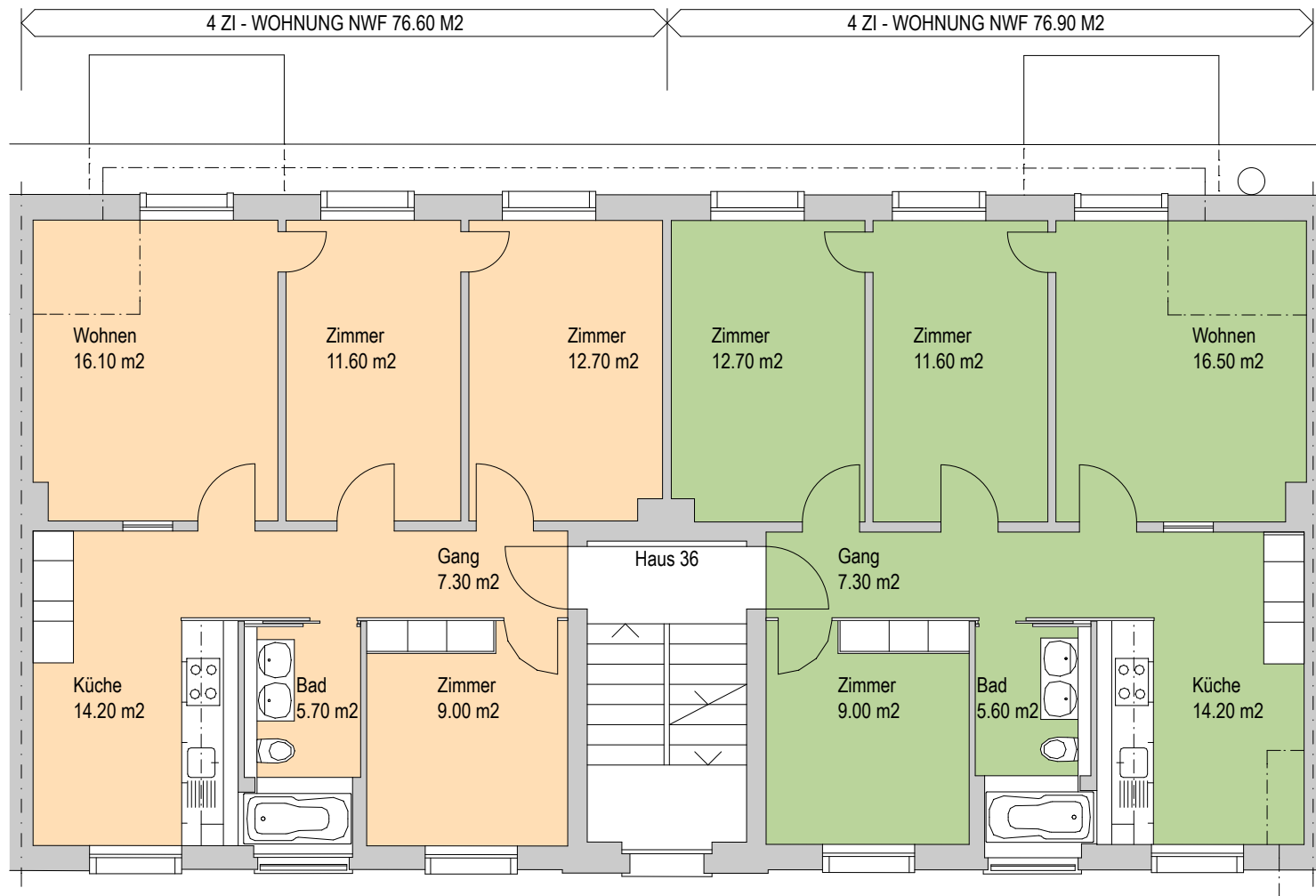
5. OBERGESCHOSS 1 : 100 NWF = NETTOWOHNFLÄCHE
