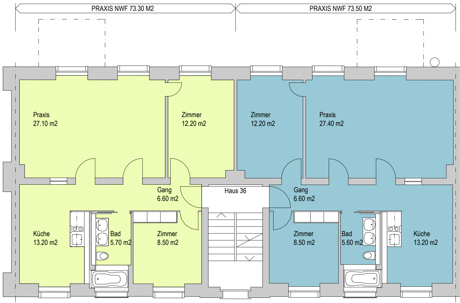
ERDGESCHOSS 1 : 100 NWF = NETTOWOHNFLÄCHE
