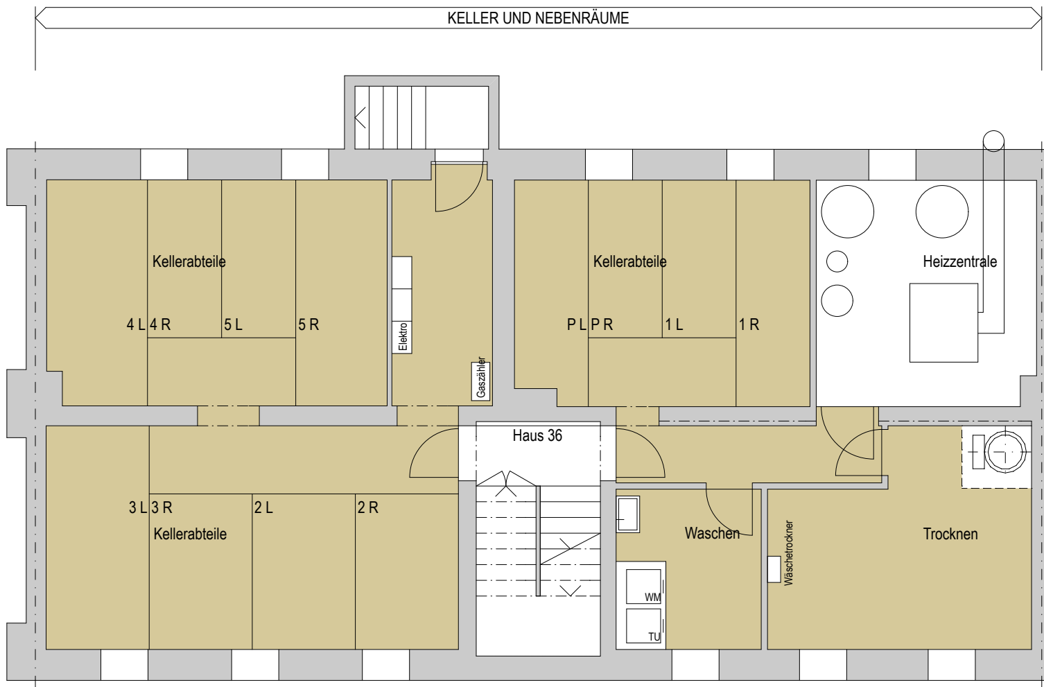
KELLERGESCHOSS 1 : 100
