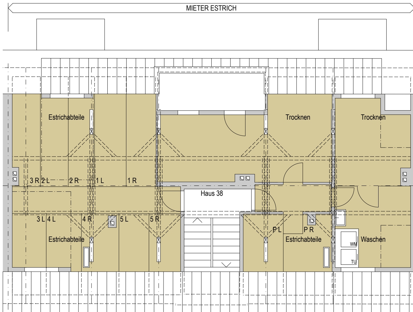
DACHGESCHOSS 1 : 100
