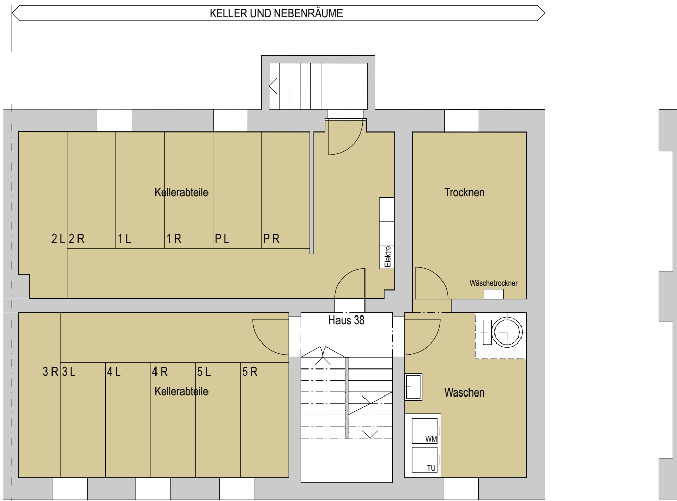
KELLERGESCHOSS 1 : 100
