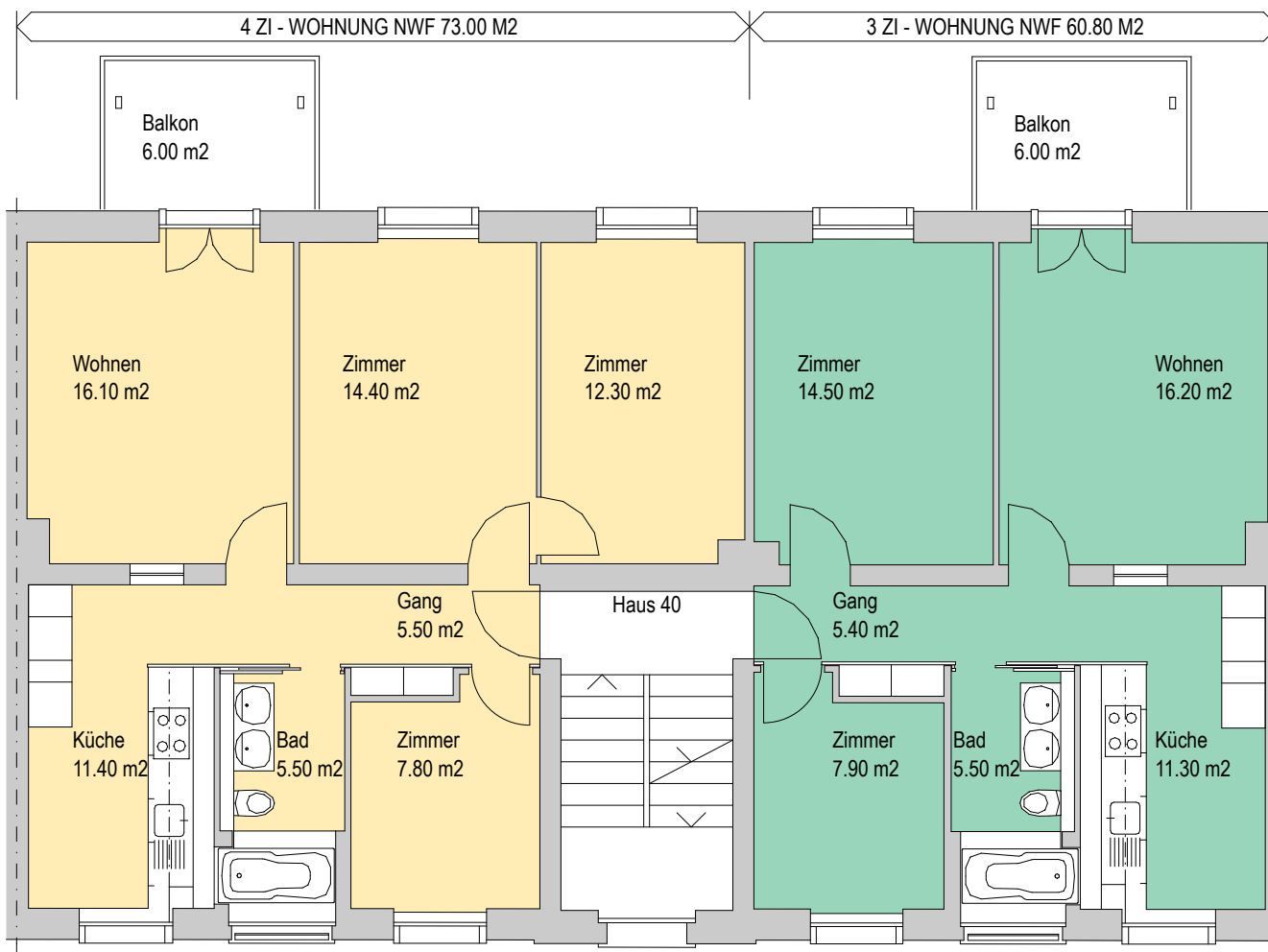
1. - 4. OBERGESCHOSS 1 : 100 NWF = NETTOWOHNFLÄCHE
