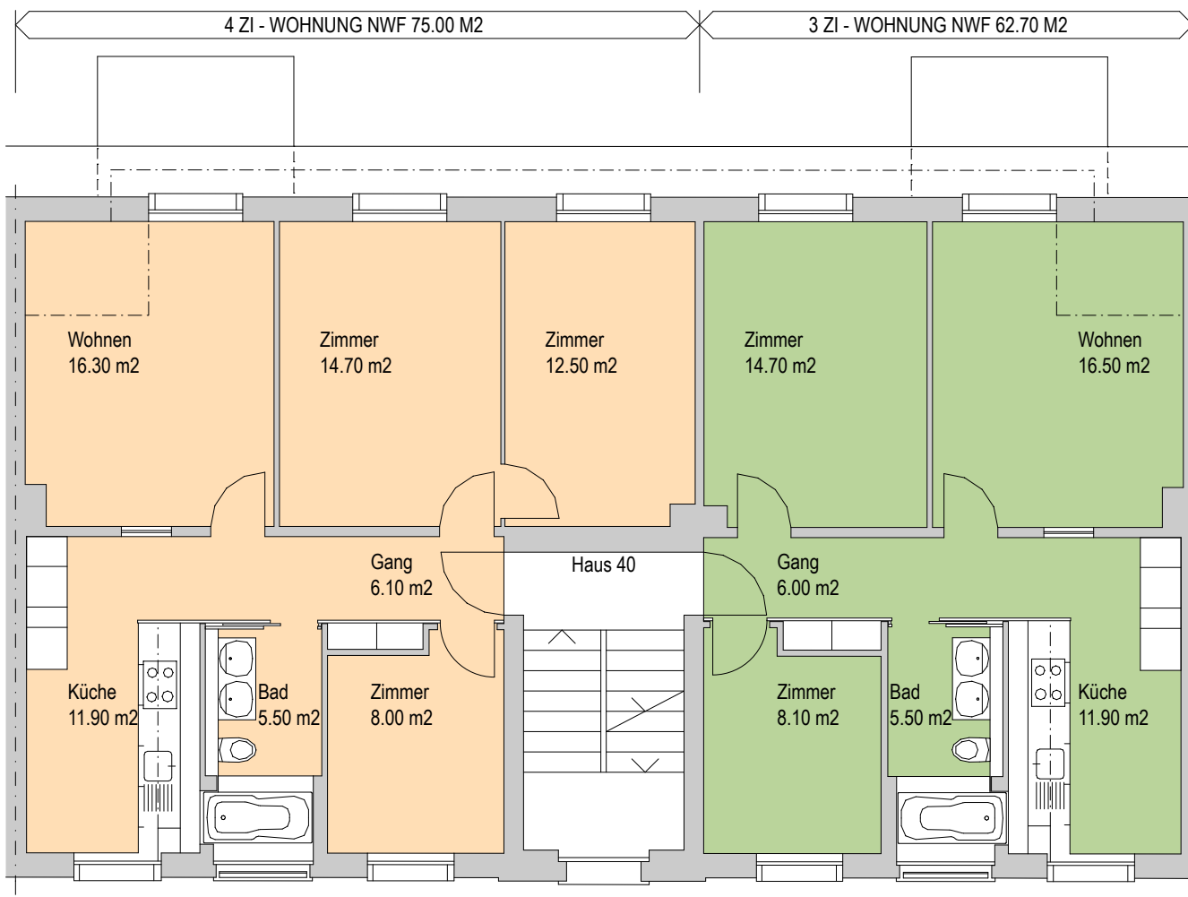
5. OBERGESCHOSS 1 : 100 NWF = NETTOWOHNFLÄCHE
