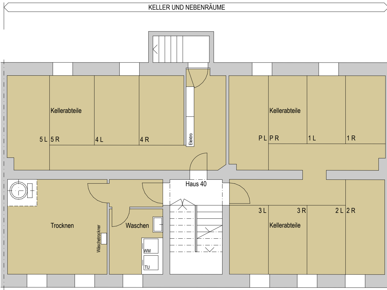
KELLERGESCHOSS 1 : 100
