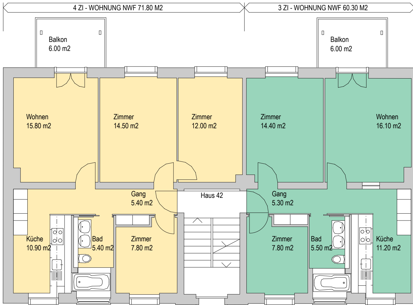
1. - 4. OBERGESCHOSS 1 : 100 NWF = NETTOWOHNFLÄCHE
