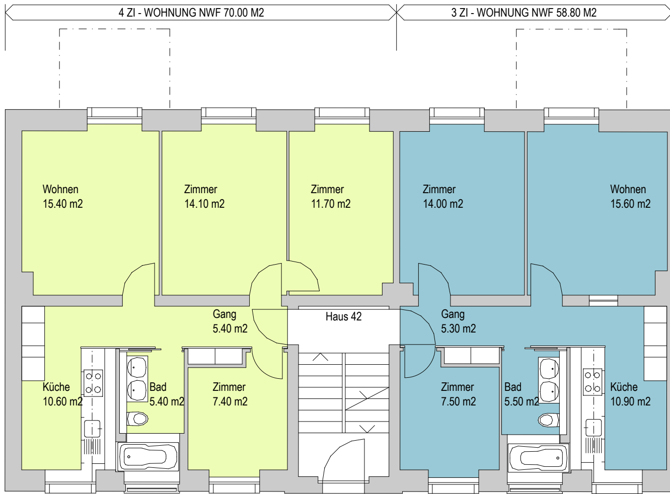
ERDGESCHOSS 1 : 100 NWF = NETTWOHNFLÄCHE
