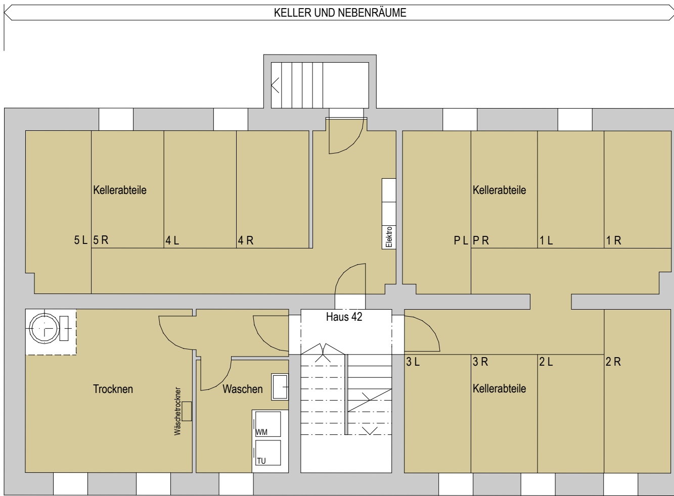
KELLERGESCHOSS 1 : 100
