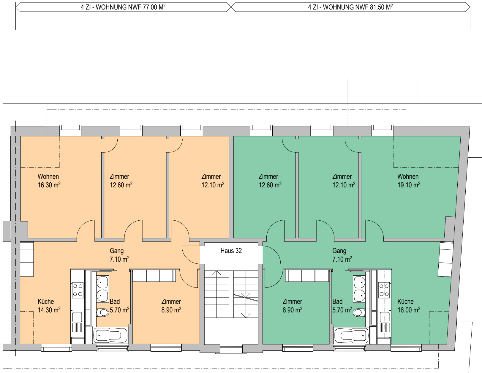
5. OBERGESCHOSS 1 : 100 NWF = NETTOWOHNFLÄCHE
