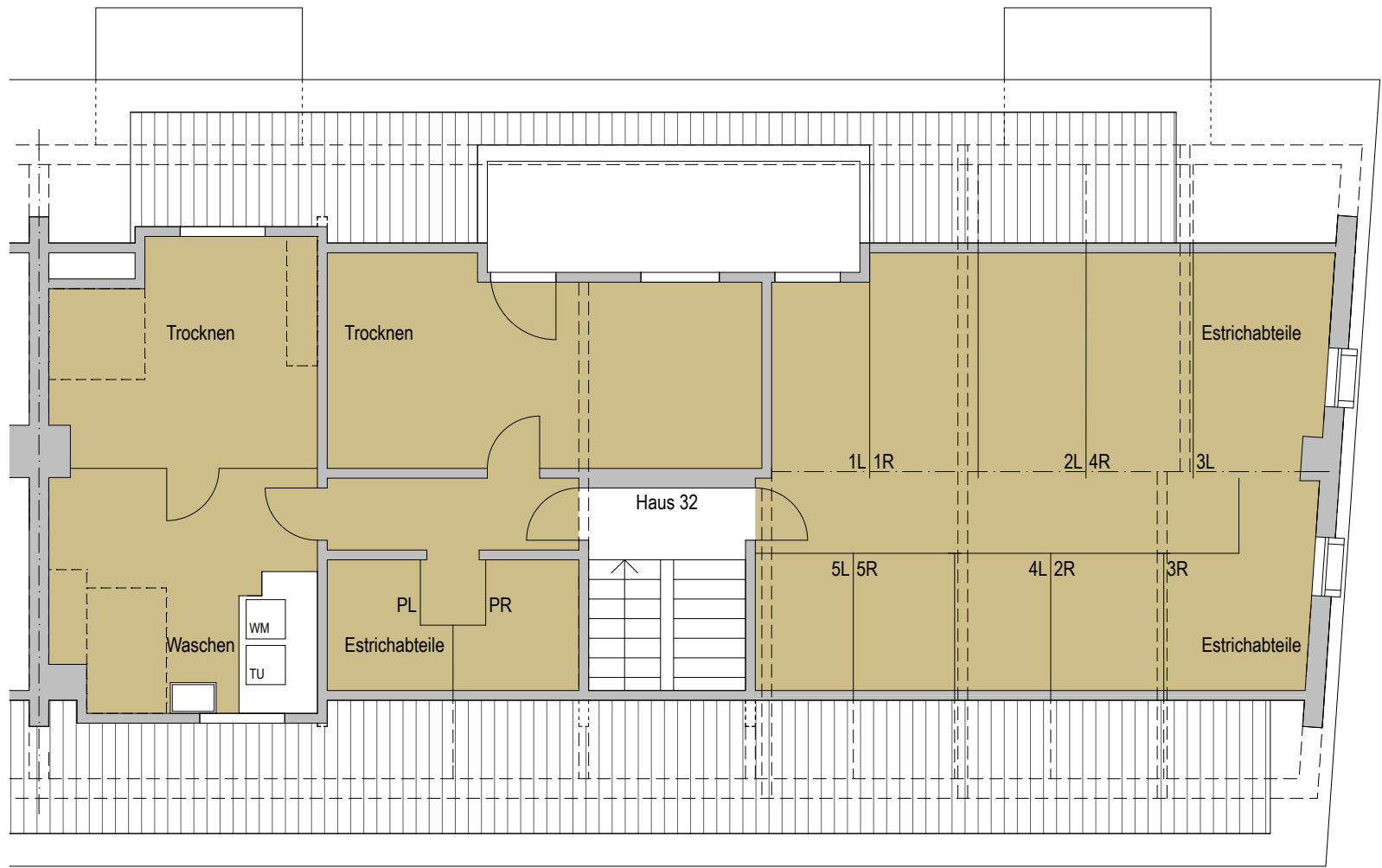
DACHGESCHOSS 1 : 100
