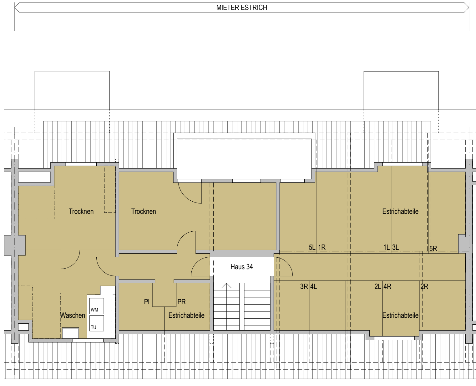
DACHGESCHOSS 1 : 100
